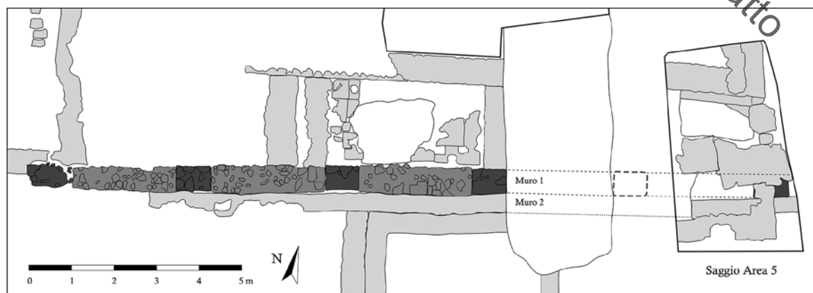
Fig. 13 - Saggio di scavo e dettaglio settore ovest: in evidenza i pilastri, sulla destra in tratteggio l'ipotetica collocazione del pilastro ancora interrato sotto il risparmio di terreno.
