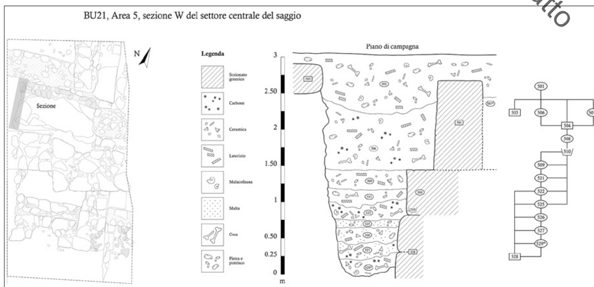
Fig. 10 - Sezione ovest del settore centrale del saggio e relativo matrix (Area 5).
