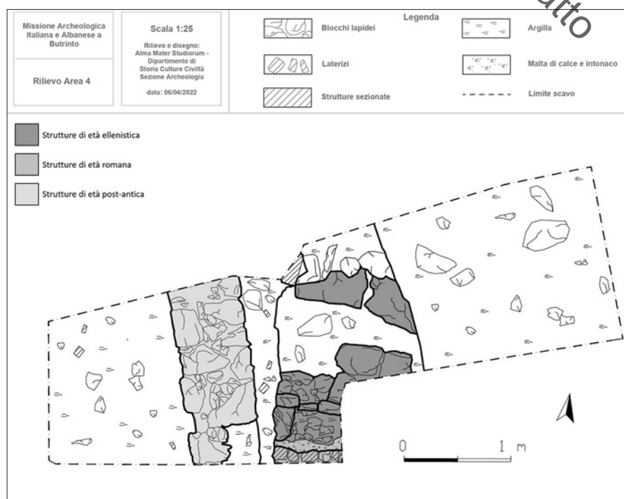
Fig. 7 - Pianta generale di Area 4 con le principali fasi cronologiche.
