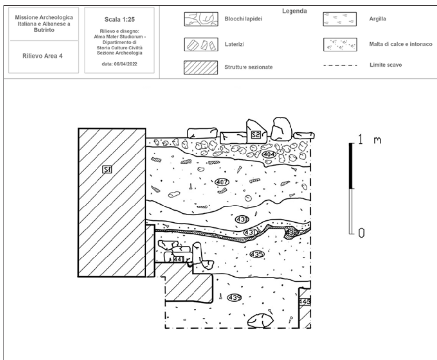
Fig. 8 - Sezione ovest del saggio (Area 4).
