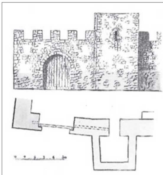
Fig. 17. Ipotesi ricostruttiva del prospetto e pianta della torre nord-orientale e della porta (da BAÇE 1976, p. 58, fig. 20).
