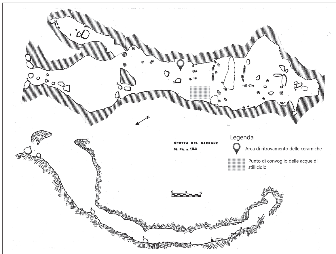
Fig. 7 - Grotta del Garrone, rilievo speditivo del 1986: pianta e sezione longitudinale (rielaborazione, da MANNINO 2017, fig. 2).
