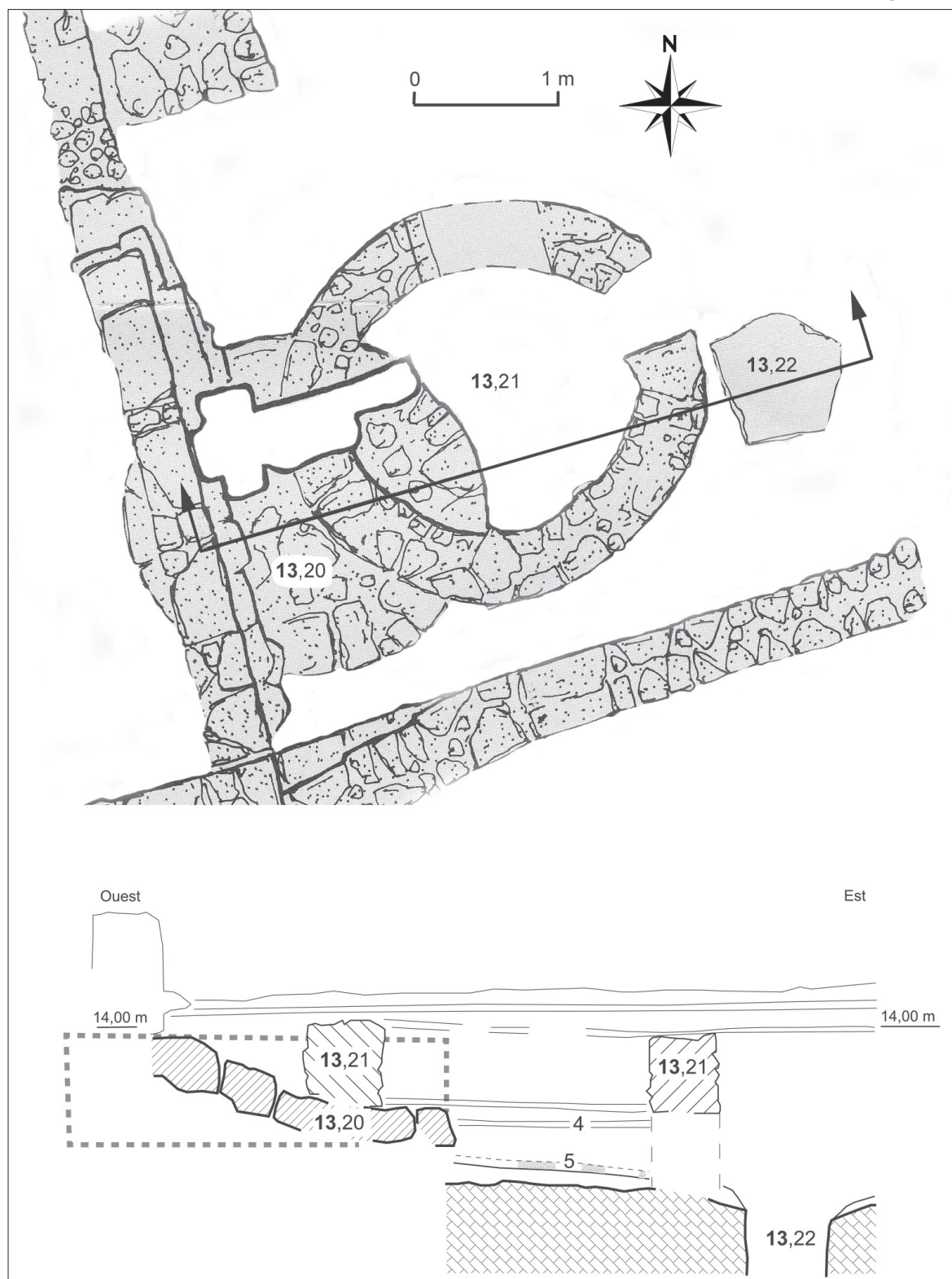
Fig. 4 a-b - Piattaforma 13,20, pianta e sezione, modificato da Megara 1 e Megara 5 fig. 463.
