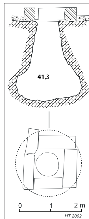
Fig. 3 - Pianta e sezione del silos 41,3 a Nord-Est dell'agorà (da Megara 5).
