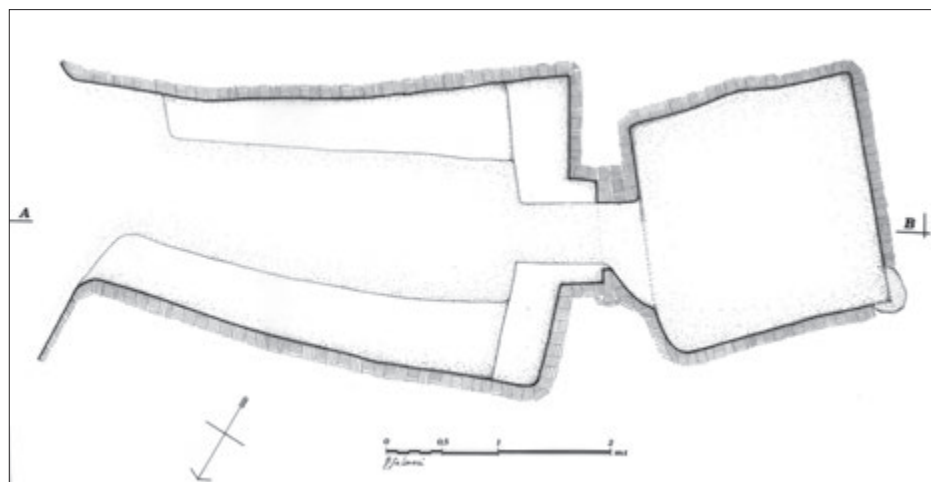
Fig. 3 – Cava Ruccia. Pianta della tomba 1 (rilievo di B. Salmeri).
