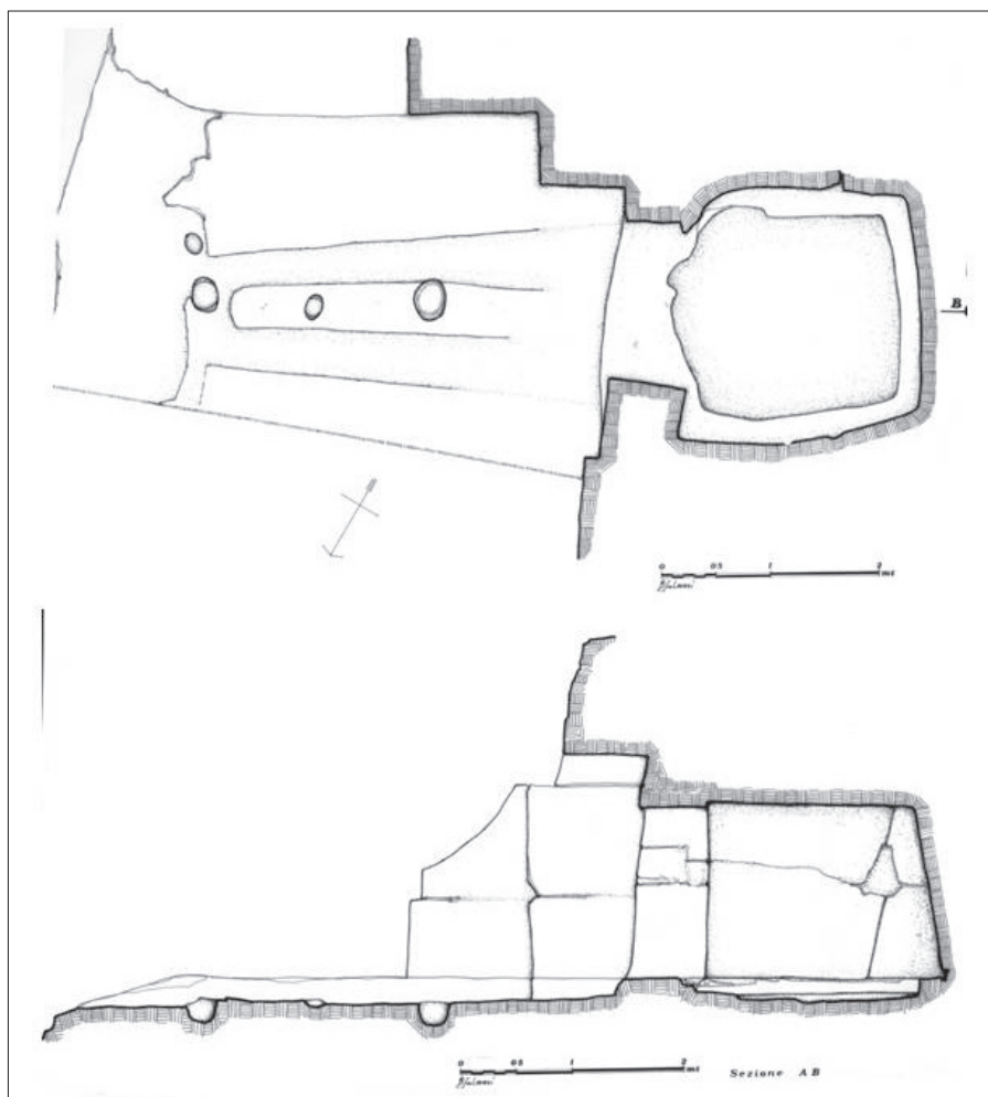
Fig. 31 – Cava Ruccia. Pianta e sezione della tomba 6 (rilievo di B. Salmeri).
