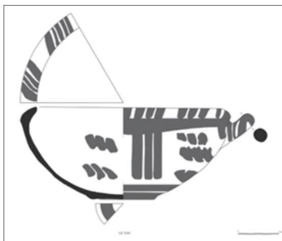
Fig. 16 – Cava Ruccia. Scodella n. 5,8 (disegno di S. Arrabito).
