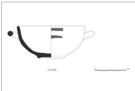
Fig. 34 – Cava Ruccia. Coppa n. 8,1 (disegno di S. Arrabito).
