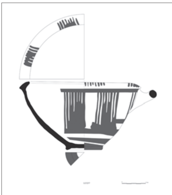
Fig. 25 – Cava Ruccia. Scodellone n. 5,17 (disegno di S. Arrabito).
