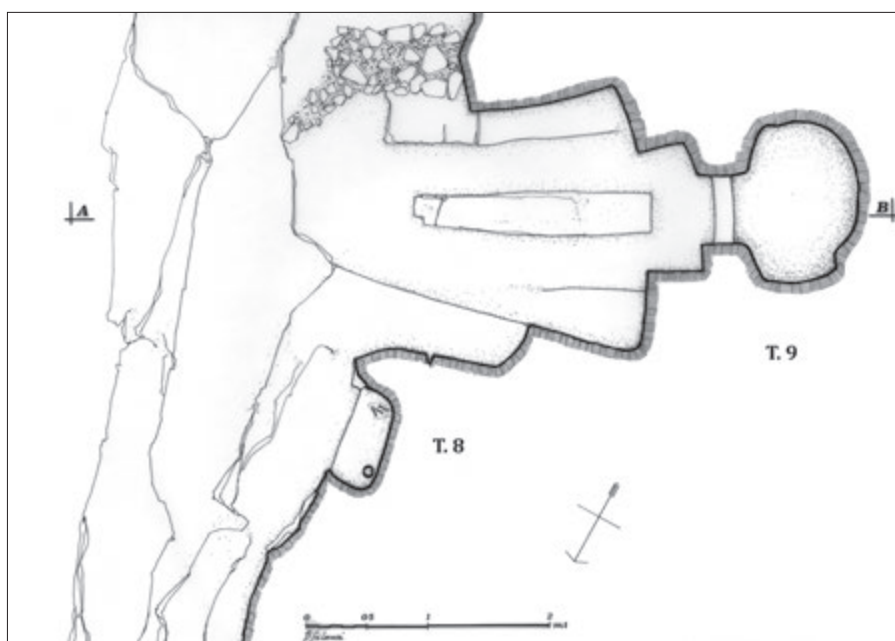
Fig. 32 – Cava Ruccia. Pianta delle tombe 8 e 9 (rilievo di B. Salmeri).
