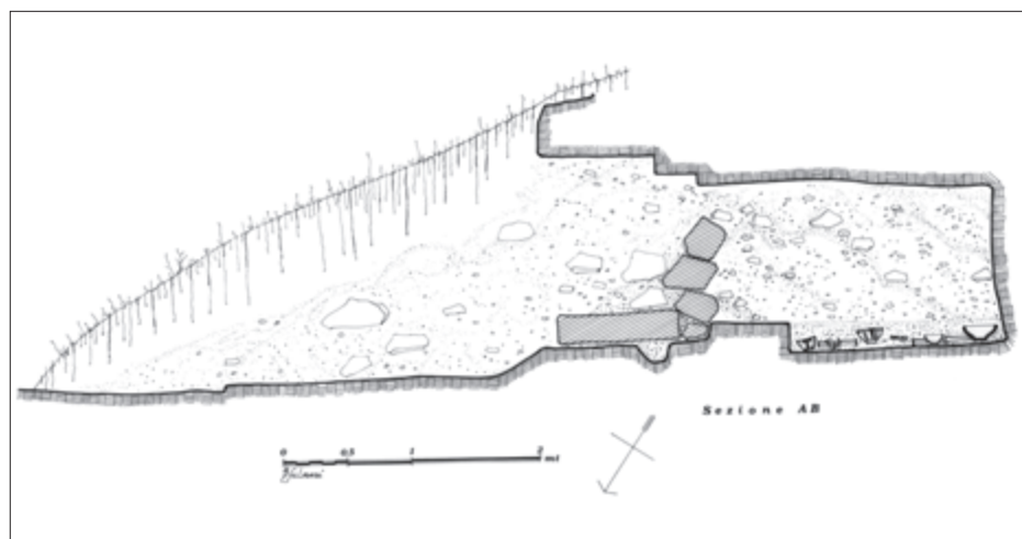
Fig. 5 – Cava Ruccia. Sezione della tomba 5 (rilievo di B. Salmeri).
