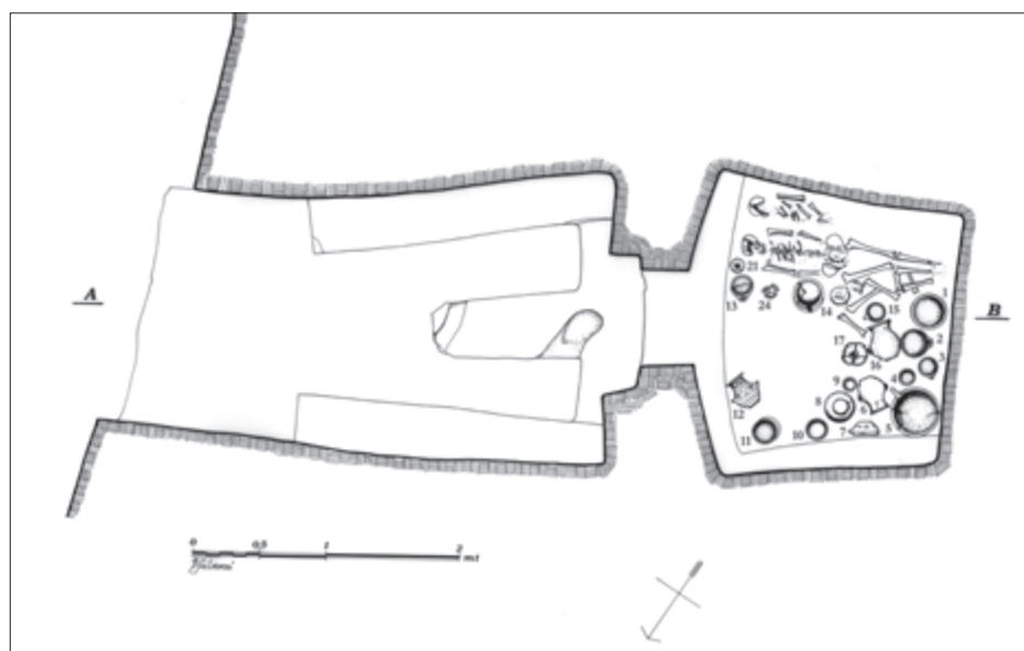
Fig. 4 – Cava Ruccia. Pianta della tomba 5 (rilievo di B. Salmeri).
