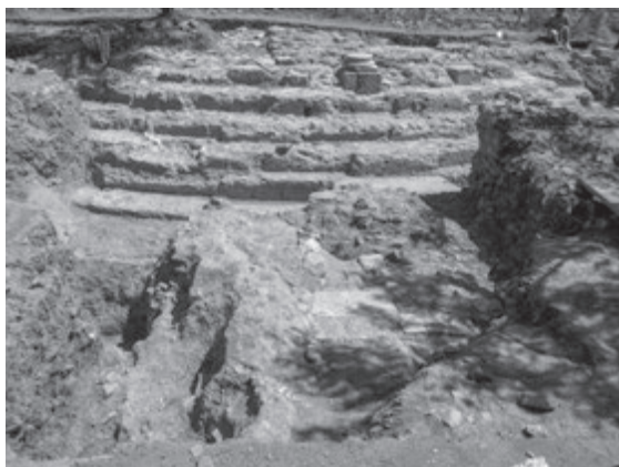
Fig. 6. Edificio III dettaglio della crepidine. In primo piano il nucleo in cementizio del monumento II (foto dell'A.).
