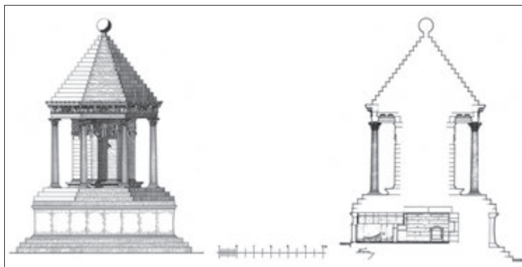
Fig. 25. Efeso. Ottagono: ricostruzione dell'elevato e sezione (da THÜR 1990).
