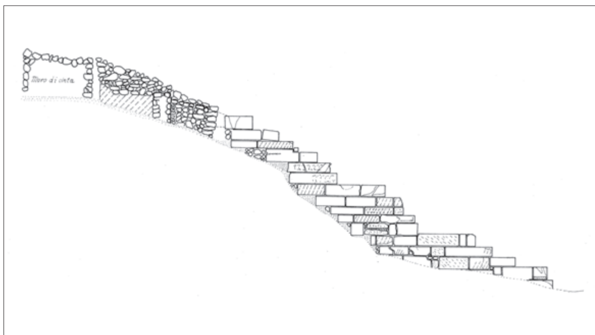
Fig. 8. Montagna di Marzo. Rilievo della torre sud, lato ovest.
