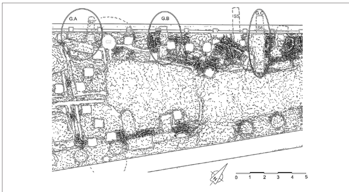
Fig. 2 - Licodia Eubea. Planimetria dello scavo del 1991 (Soprintendenza BB.CC.AA. di Catania; Dis. arch. Sebastiano Ragusa. Rielaborazione grafica di Irene Novello e Andrea Raiti).
