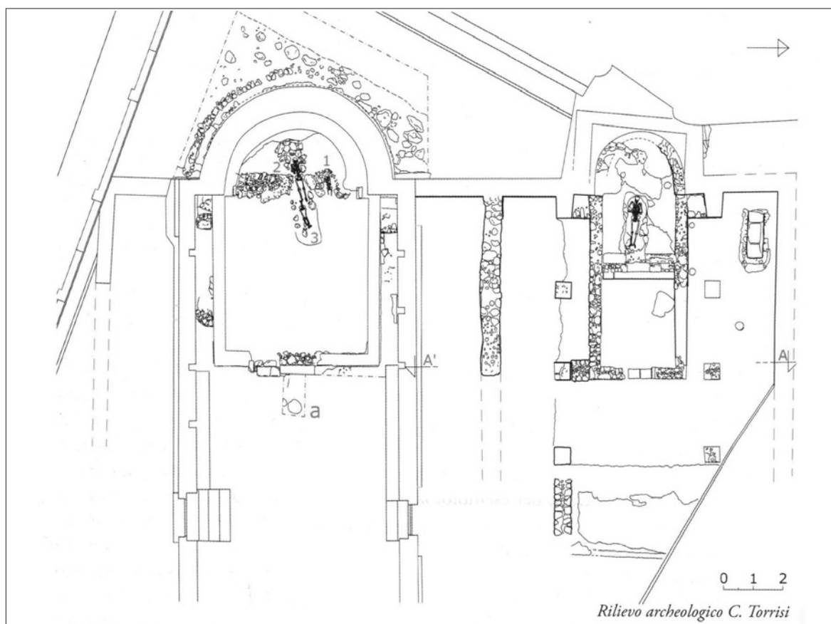
Fig. 10 - Planimetria dell'area della Nunziatella dopo lo scavo (TAORMINA 2015, p. 106, fig. 14).
