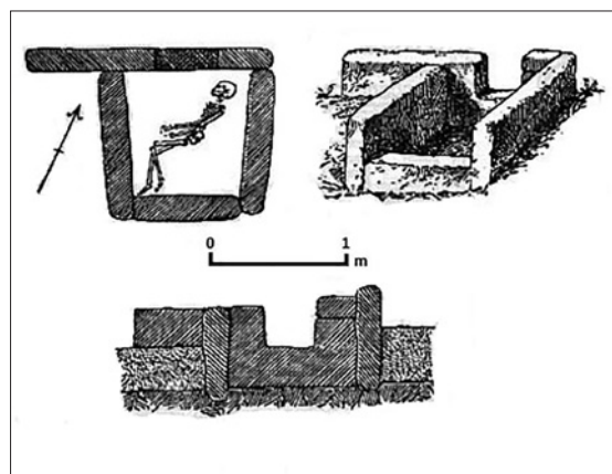
Fig. 24 - Monte Racello. Tomba 8. Planimetria e sezione (da Orsi 1898, fig. 13).
