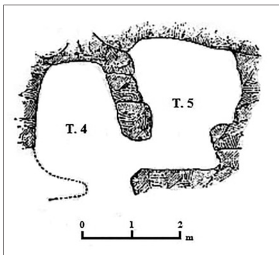
Fig. 13 - Monte Racello. Tomba 4 e 5. Planimetria (rielaborata da Orsi 1898, fig. 11).
