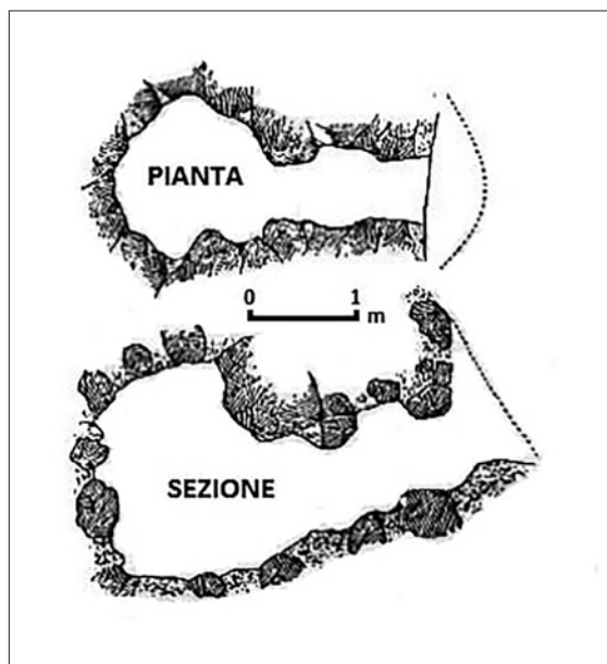
Fig. 23 - Monte Racello. Tomba 6. Planimetria e sezione (rielaborata da Orsi 1898, fig. 12).
